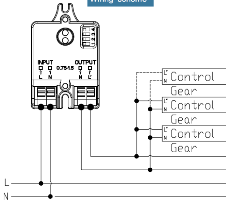
Wiring scheme
